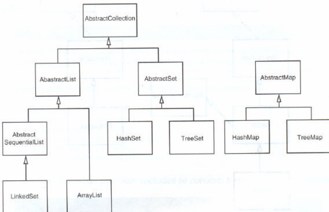
Figura 2.14 Estructura de clases de colecciones. Está formada por:
